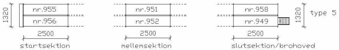
Plan af FLEX-BADEBRØ (dobbelt) med adgangstrin, gelønder og alu-stige
