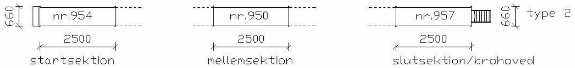
Plan af FLEX-BADEBRØ (enkelt) med adgangstrin, gelønder og alu-stige
